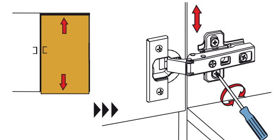
Réglage en hauteur Vertical adjustment
